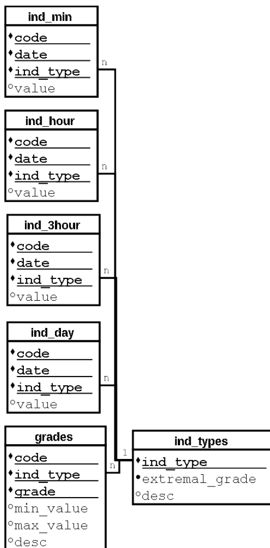
Рисунок 5 – Схема таблиц для хранения информации об индикаторах геомагнитной активности
