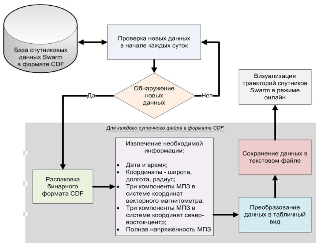
Рисунок 3 – Блок-схема автоматизированной загрузки данных спутников Swarm
