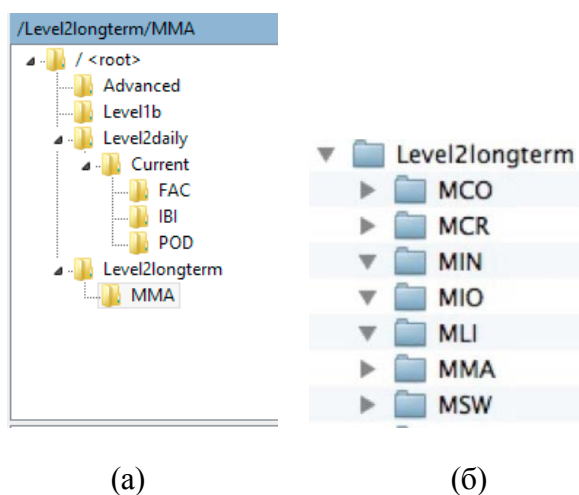
Рисунок 2 – Содержание каталога долговременных данных уровня 2 (Level2longterm) на данный момент (а) и предполагаемое его содержание по состоянию на конец 2015 г. согласно справочному изданию [Swarm PDGS Data Access User Manual, 2014] (б)
