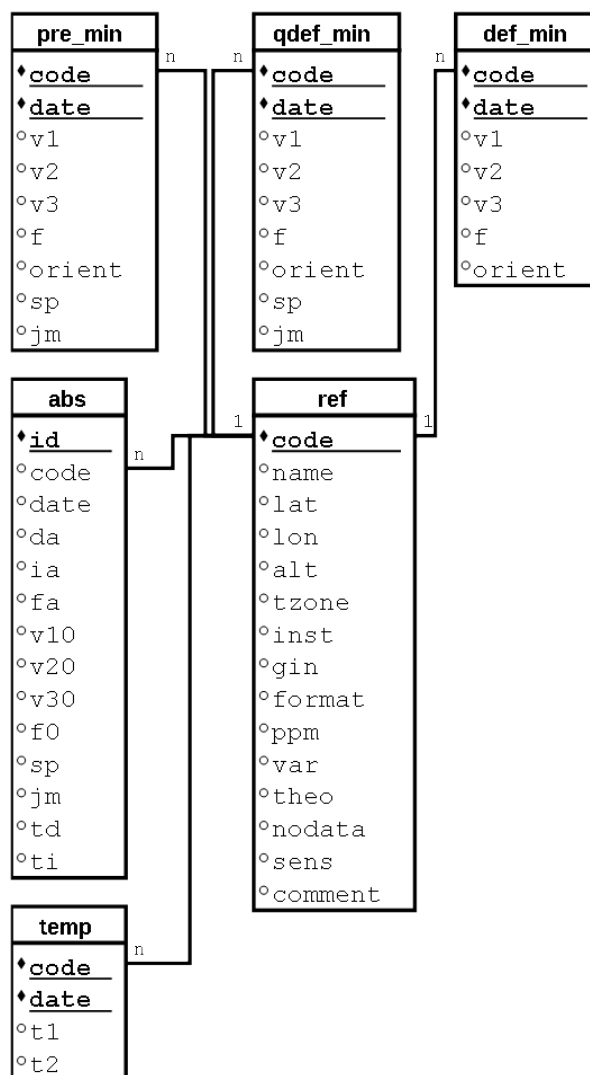
Рисунок 4 – Схема таблиц для хранения данных измерений компонент магнитного поля Земли. В таблицах pre_min, qdef_min и def_min хранятся минутные предварительные, квазиокончателные и окончательные данные соответственно
