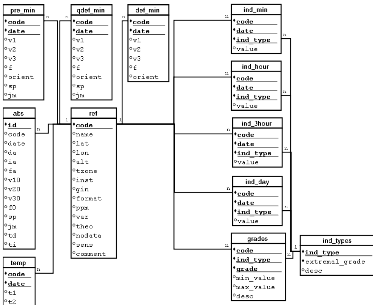
Рисунок 6 – Общая схема базы данных
