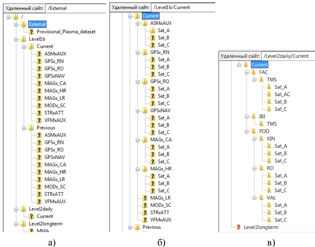
Рисунок 1 – Структура корневого каталога (а), директории «Level-1b Current» (б), директории «Level2daily Current» (в) на сервере ЕКА
